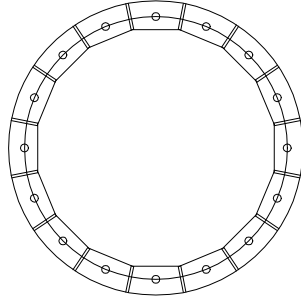
TEPE FLANŞI TOP PLATE
